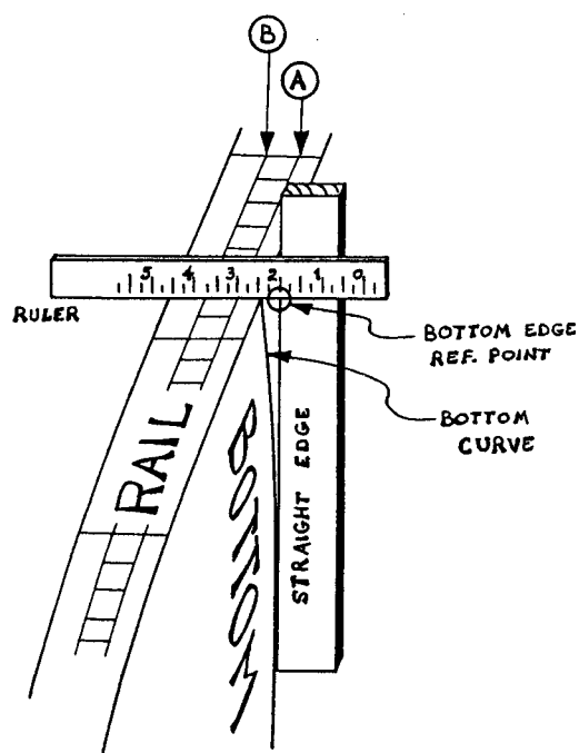
FIG. 6-14 BOTTOM EDGE REFERENCE POINT
