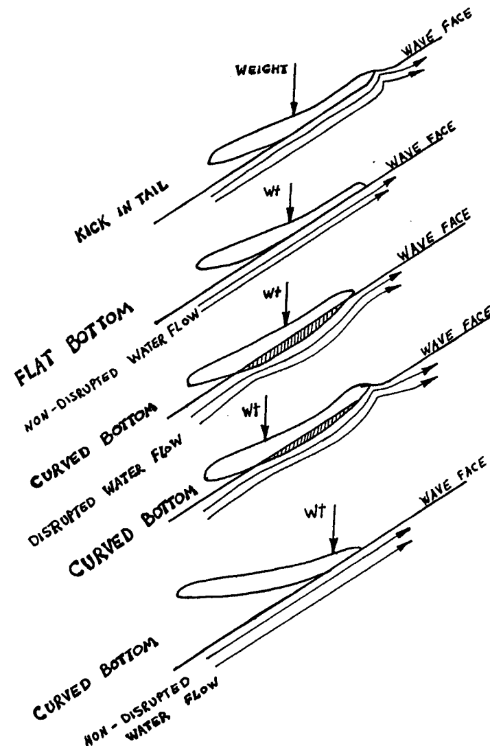
FIG. 2-5 BOTTOM ROCKER
